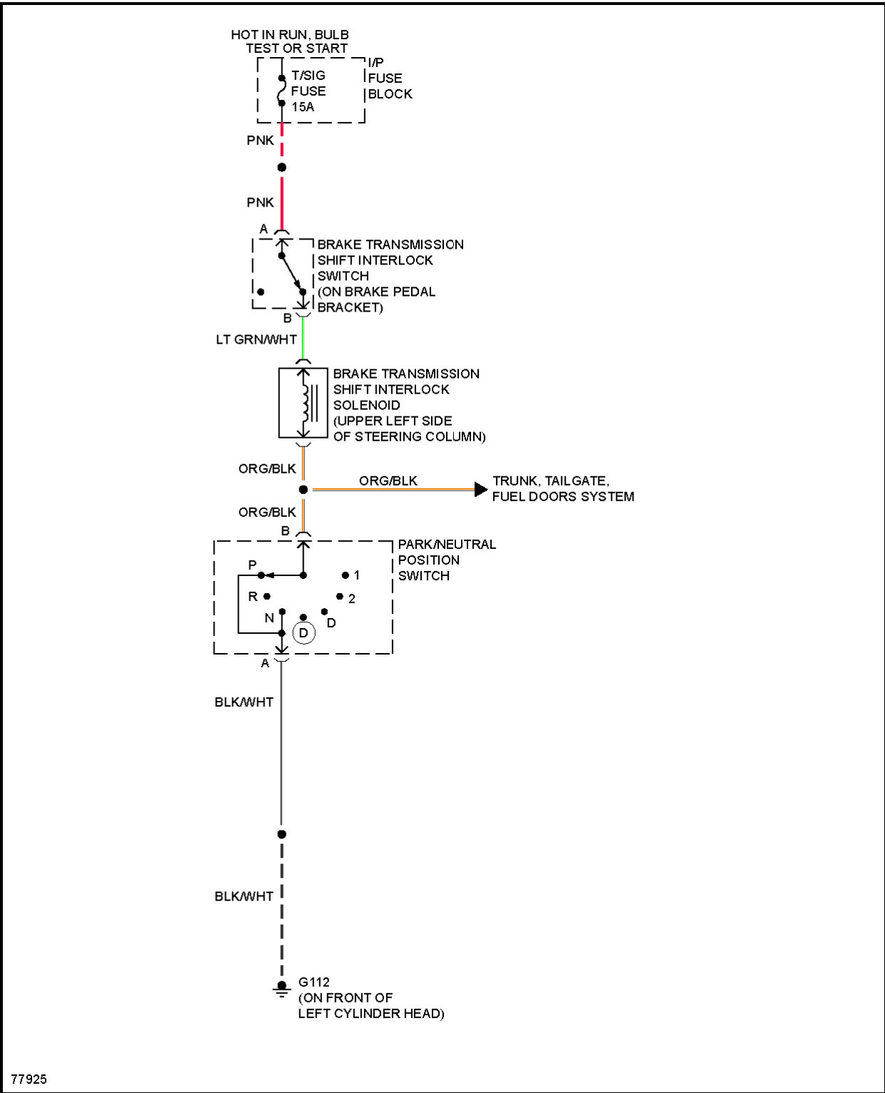
Fig. 36: Shift Interlock Circuit
