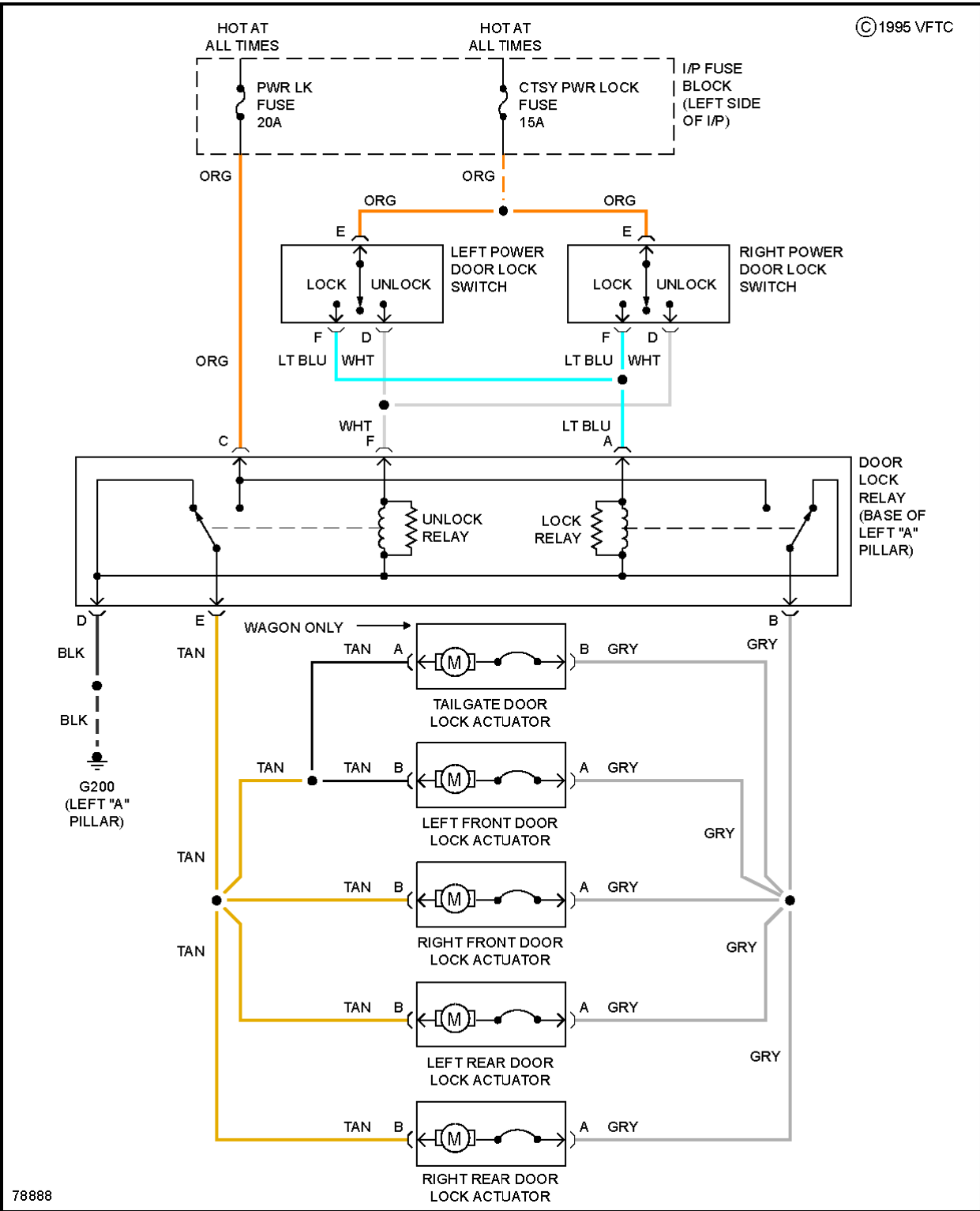
Fig. 31: Door Lock Circuit
